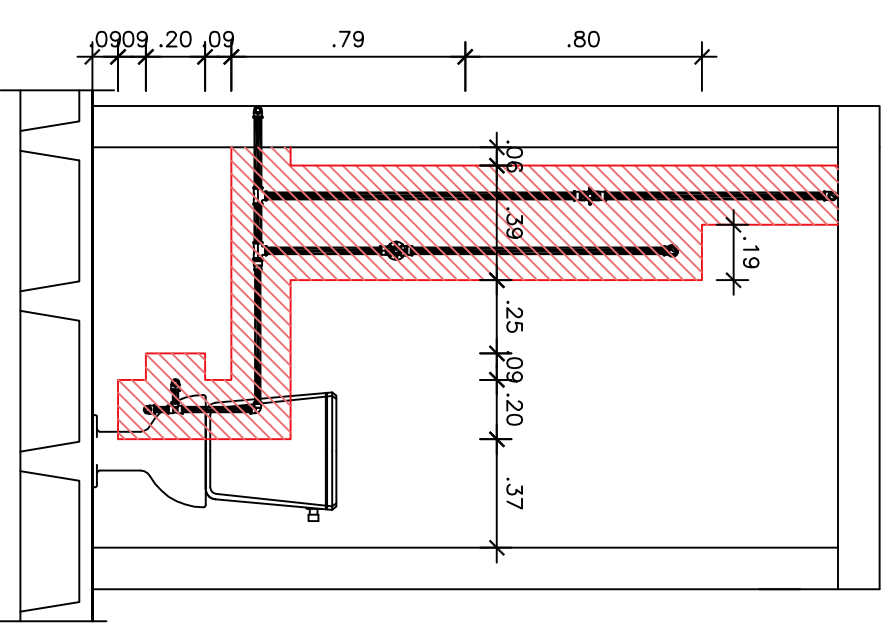
Vista D ESCALA 1/25
