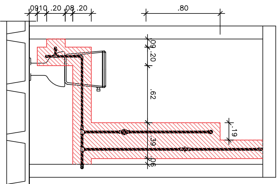
Vista A ESCALA 1/25
