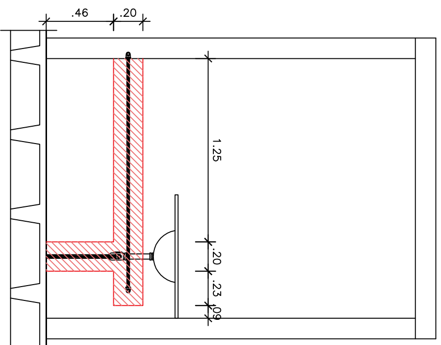
Vista B ESCALA 1/25
